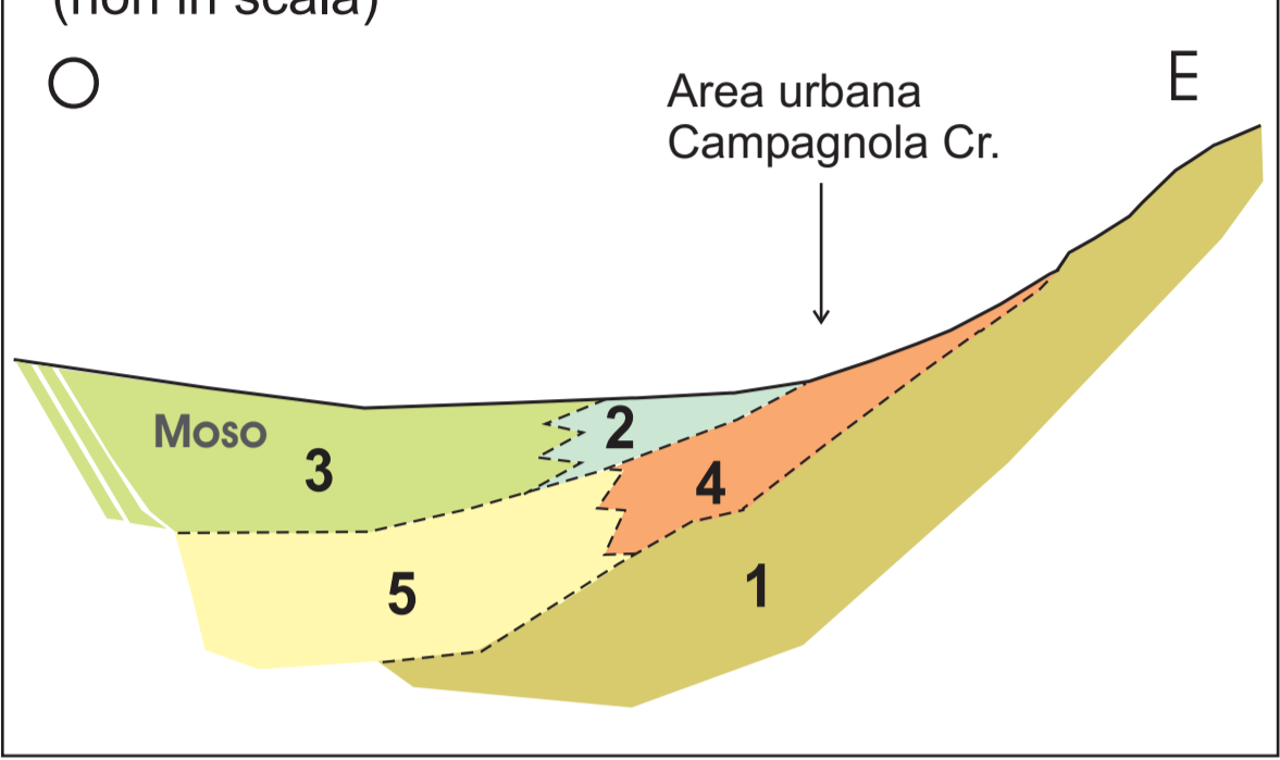
Schema deposizionale unità geomorfologiche (non in scala)
